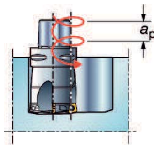
Spiralinterpolation bei hohem Vorschub
