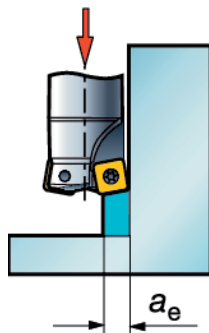
Tauchfräsen
